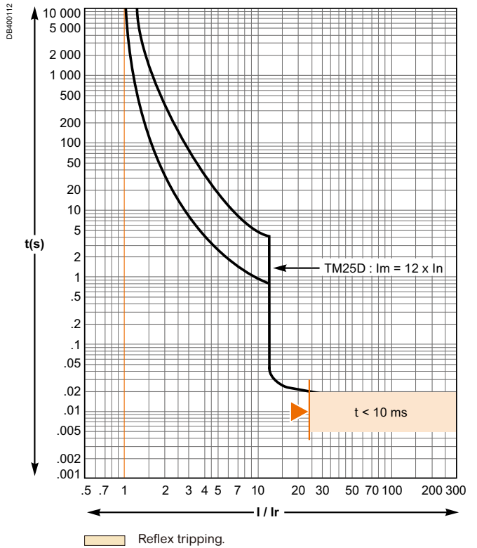
TM25D
