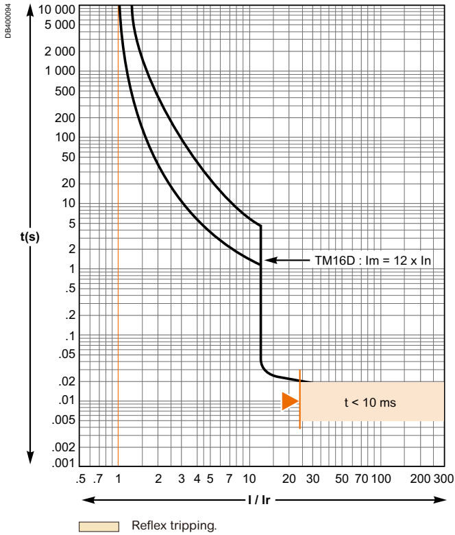
TM16D
