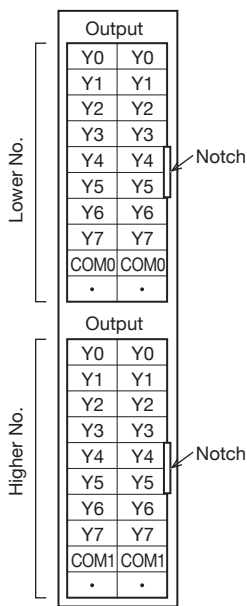
FX5-C32EYT/D
