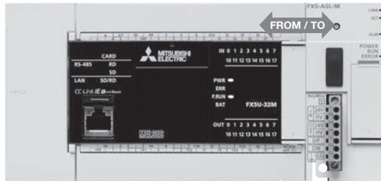
FX5-ASL-M
