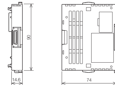
FX5-CNV-IFC
