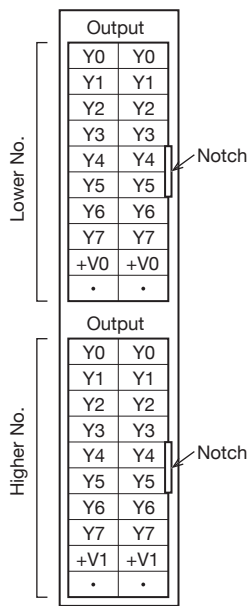
FX5-C32EYT/DSS
