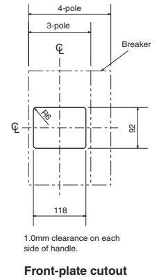
Front-plate cutout
