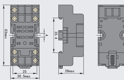
63×30.5×26(mm)
