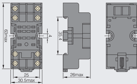
63×30.5×26(mm)
