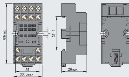
63×30.5×26(mm)
