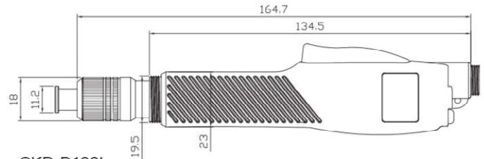
SKD-B100L
