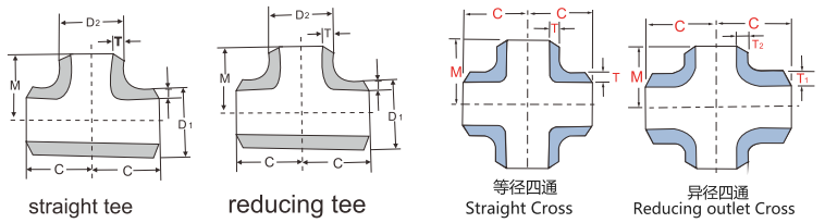
Unit:mm
